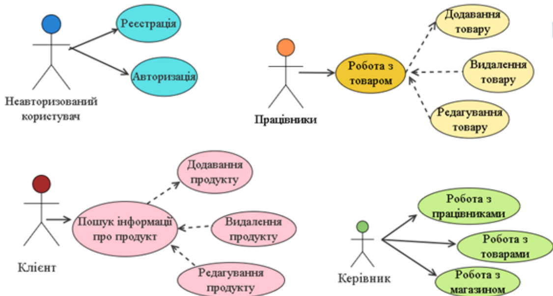
Рисунок 1 - Діаграма прецедентів використання інформаційної системи
