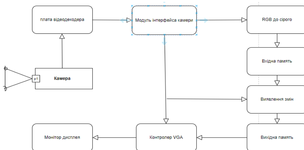
Рисунок 1 – Діаграма потоків даних процесу запису відео
