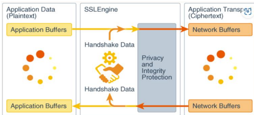
Рисунок 2. - Потік даних через JSSE
