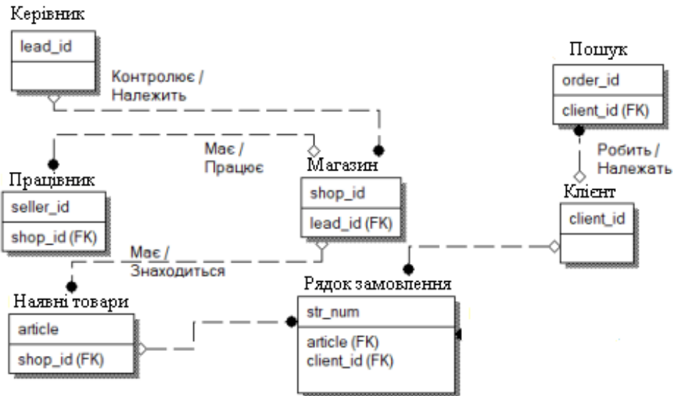
Рисунок 3 - Міграція ключів при проектуванні бази даних
