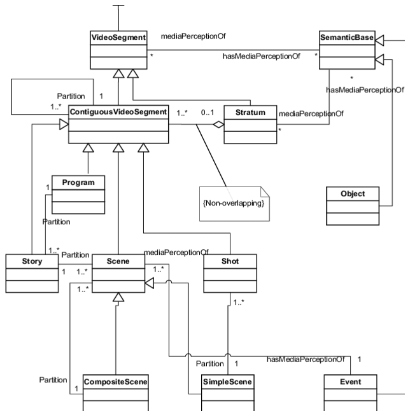
Рисунок 4 – Діаграма класів обробки відеоданих
