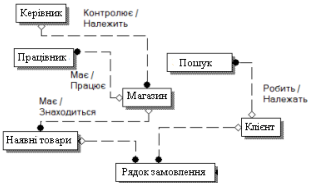
Рисунок 2 - Концептуальна модель інформаційної системи
