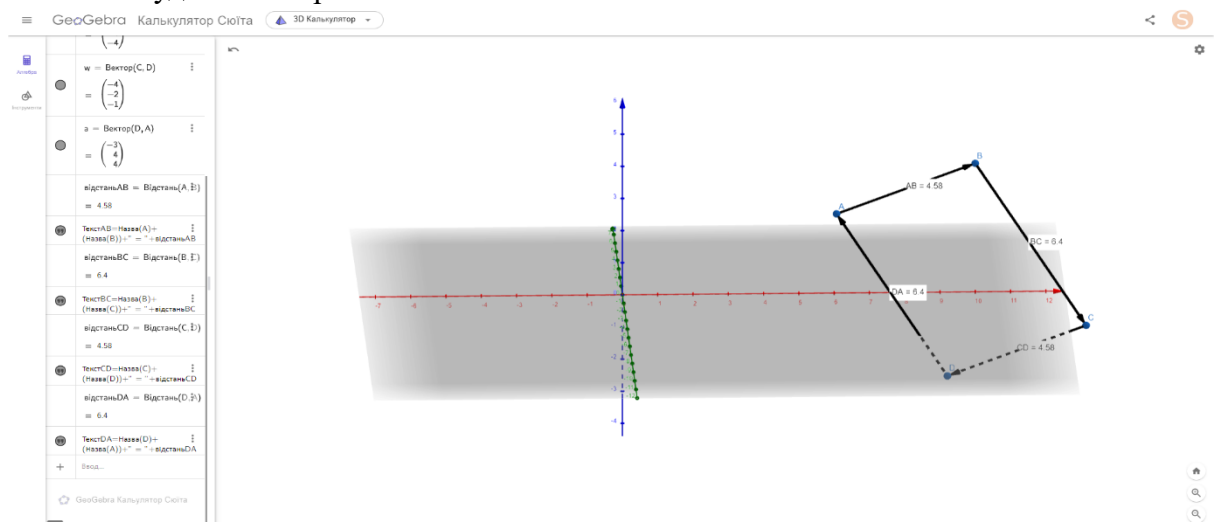
Рис. 3 Знаходження довжини
