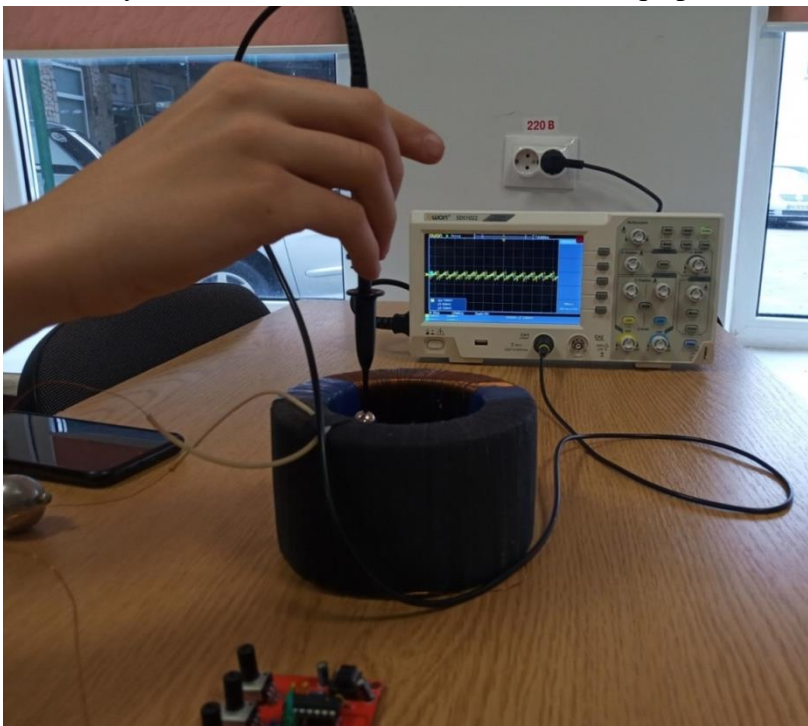
Рис. 2. Прилади для виявлення та генерації поздовжніх електричних хвиль.
