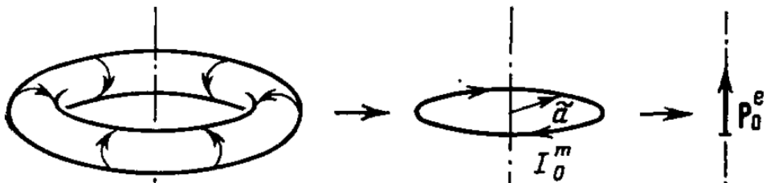
Рис. 1. Прямий соленоїд з лінійним струмом, згорнутий в тор, еквівалентний кільцевому магнітному струму, зовнішнє поле якого при стягуванні кільця в точку збігається з полем елементарного електричного диполя[1].
