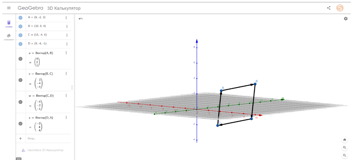
Рис. 2 Побудова векторів
