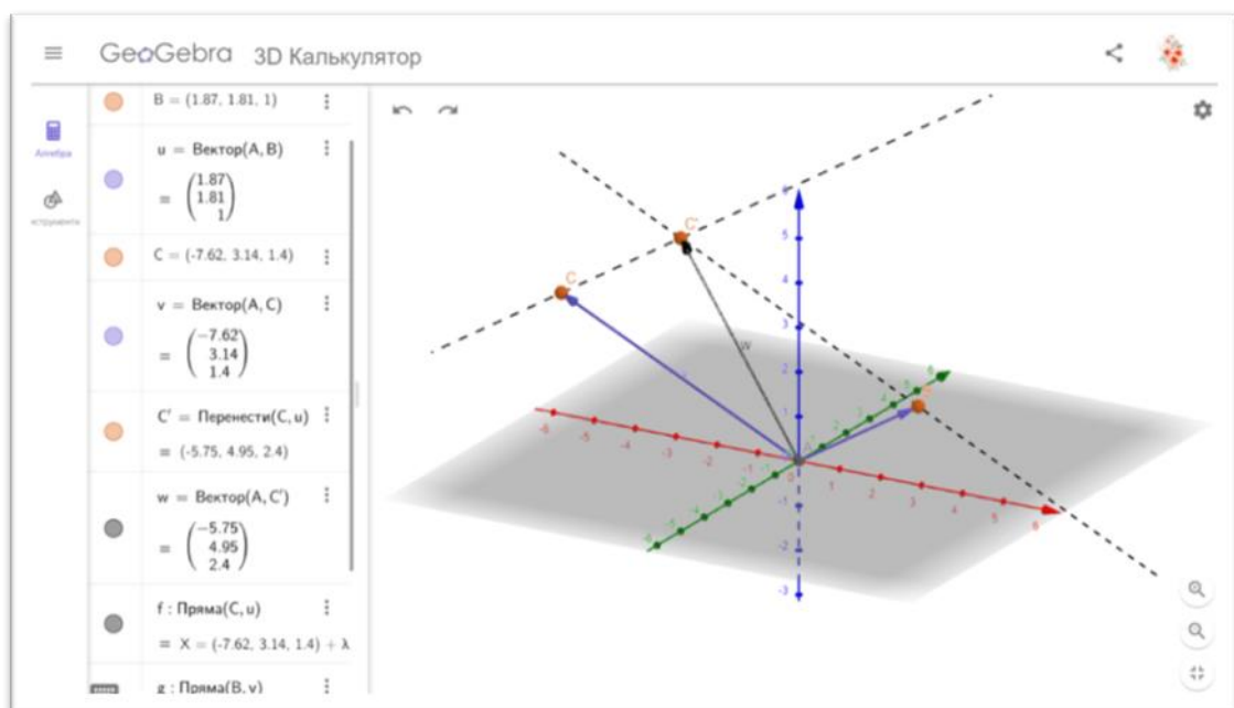
Рис. 1 Паралельне перенесення
